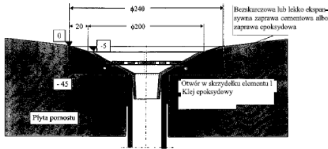
Rys. 10 Szcik sposobu osadzenia sączka - Wariant III - Etap III
