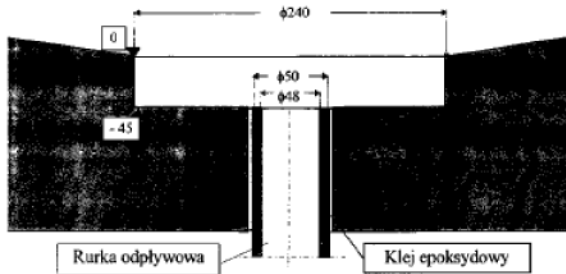
Rys. 9 Szcik sposobu osadzenia sączka - Wariant III - Etap II
